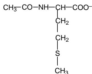
Ac-Met
